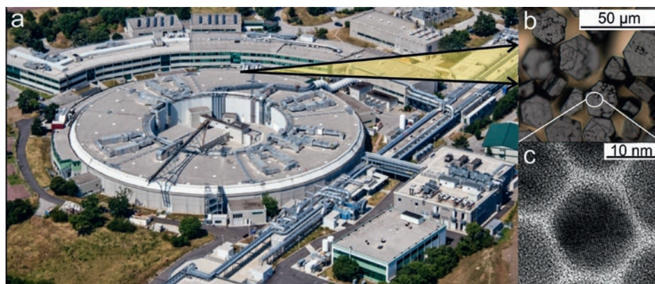
▲ Am Teilchenbeschleuniger der ETH Zürich werden Röntgenstrahlen erzeugt (a) und damit die mikrometergroßen Superkristalle bestrahlt (b). Diese bestehen aus einzelnen, regelmäßig angeordneten Nanokristallen (c).
